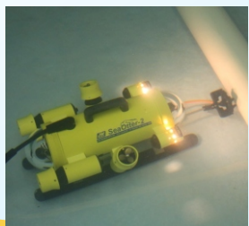
Mini ROV with UT Gauging
